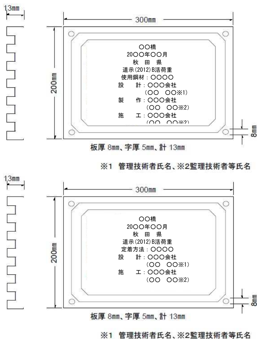
図3-2-2 銘板の寸法及び記載事項
