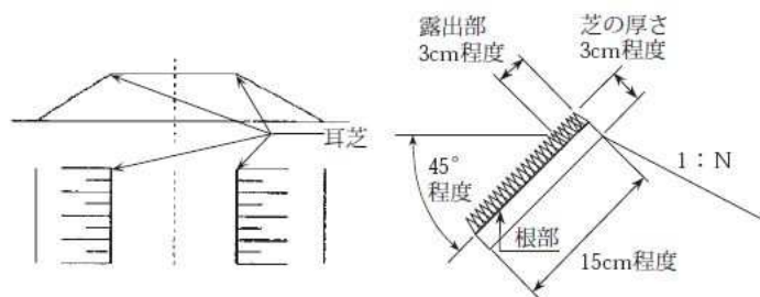
図3-2-6 耳芝
